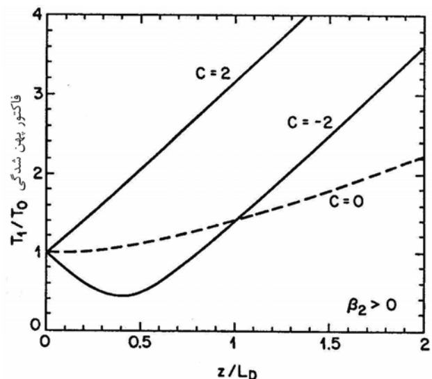
شکل ۱: ضریب پهن شدگی بر حسب تابعی از طول انتشار z/L_D ، برای پالس گوسی چرپ‌دار. نمودار خط‌چین برای پالس گوسی بدون چرپ است [۳]
